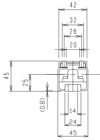
D-D断面図
