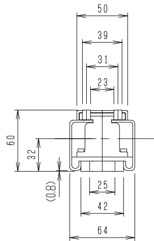
D-D断面図
