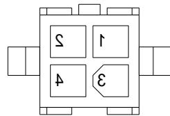
図 6.3.1.1 SIO のコネクタの端子配列
