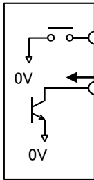
シンクタイプ PLC
