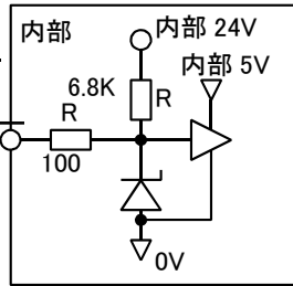
メカシリンダ入力回路
