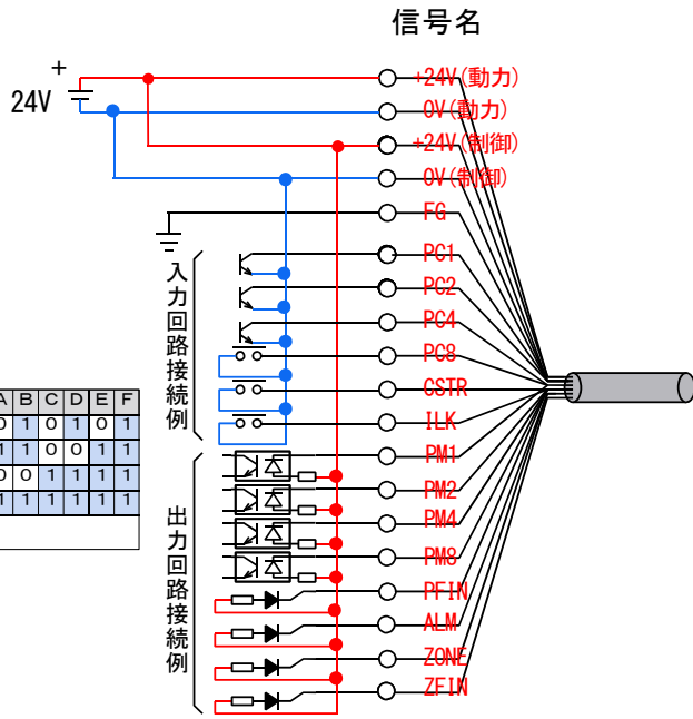
メカシリンダ出力回路
