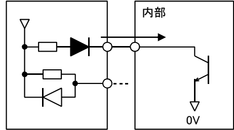
メカシリンダ出力回路
