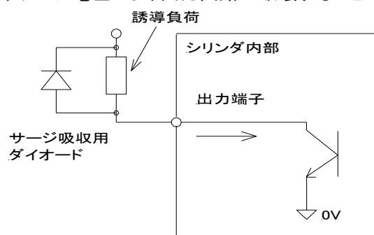
図4. メカシリンダの出力回路
