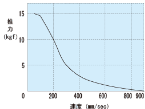
推力-速度特性
